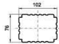
Сечение трубы
