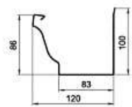
Сечение желоба
